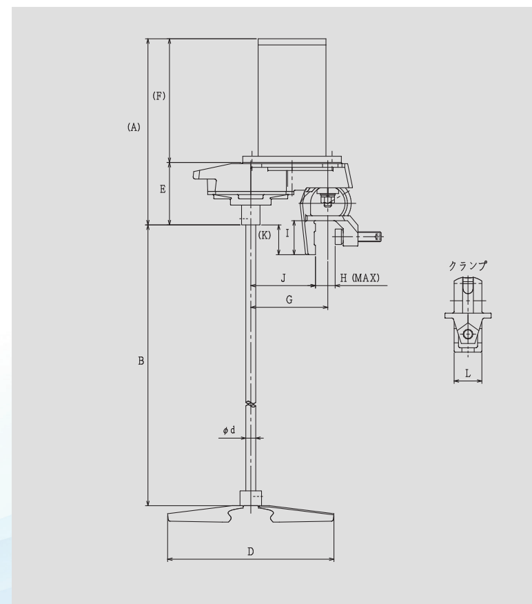
寸法図
