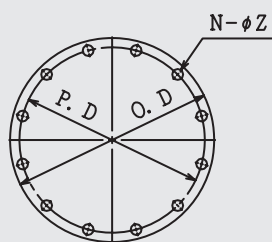
丸フランジ
