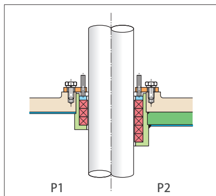
グラندパッキンシール
