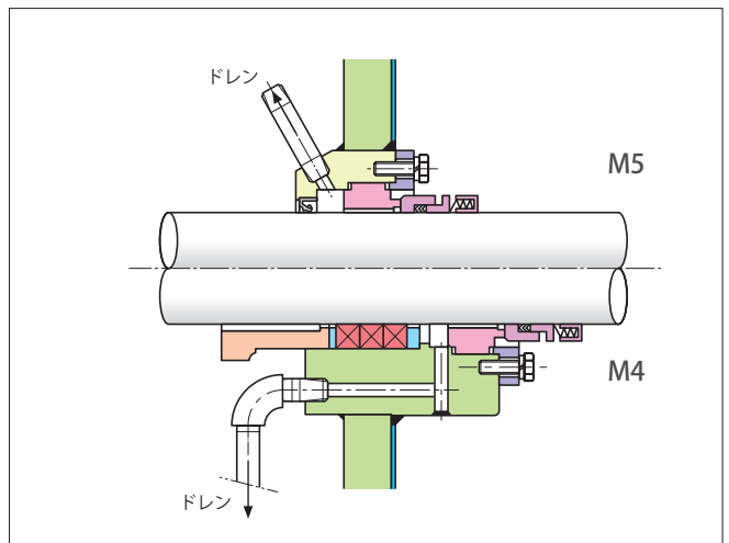
シングルメカニカルシール
