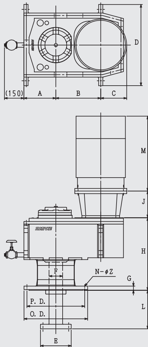
ギヤ2段・3段減速
