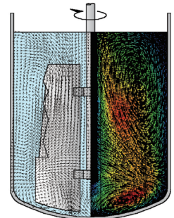
MR205 インペラのフローパターン
