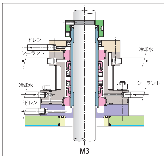
ダブルメカニカルシール
