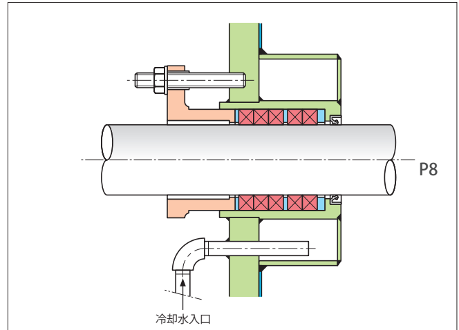
グランドパッキンシール(強制冷却)
