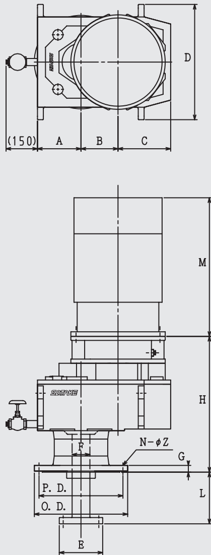
ギヤ1段減速
