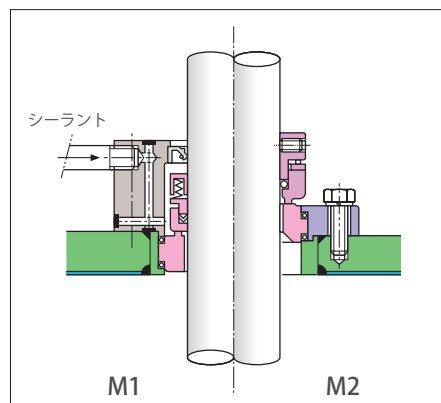
シングルメカニカルシール (真空型攪拌槽用)
