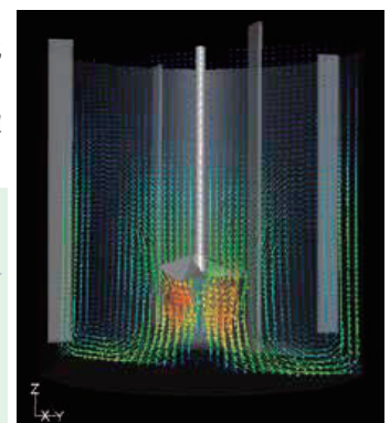
C.F.D. による数値シミュレーション結果
