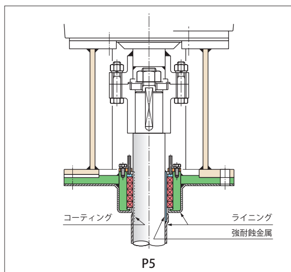
グラندパッキンシール (接液・接ガス部各種ライニング・コーティング施工)
