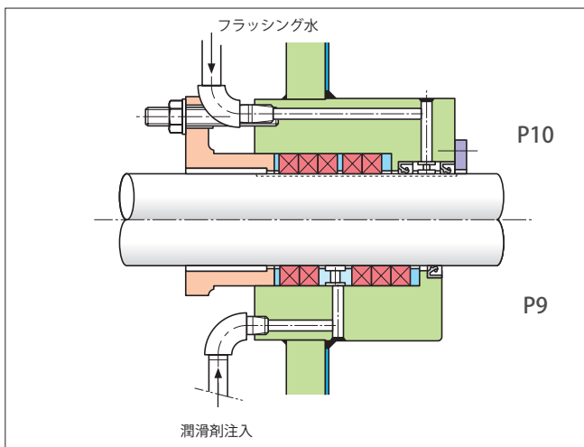
グランドパッキンシール(スラリー液対策用)
