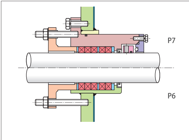
グランドパッキンシール(暫定シール方式)
